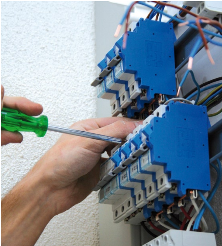
Elektroinstallation
